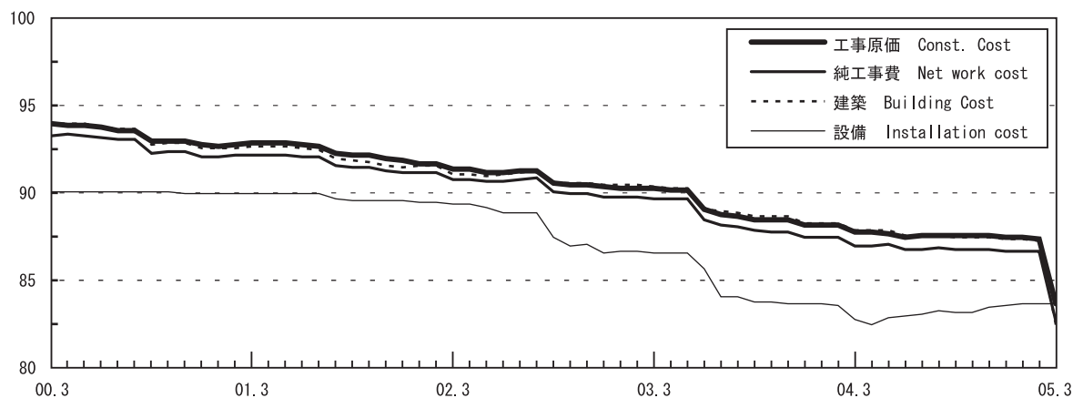
図-4 No. 32 個人住宅 W 125㎡ 平成7年平均=100 fig.4 Individual house 1995 average=100
