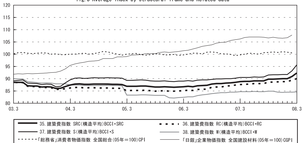
図－８ 構造別平均建築費指数(工事原価・東京)と関連統計指標との比較 fig.8 Average index by structural frame and Related data
