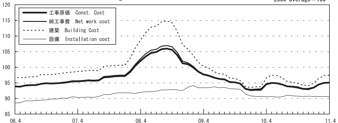
図-2 No.8 事務所 SRC 7,000㎡ fig.2 Office
