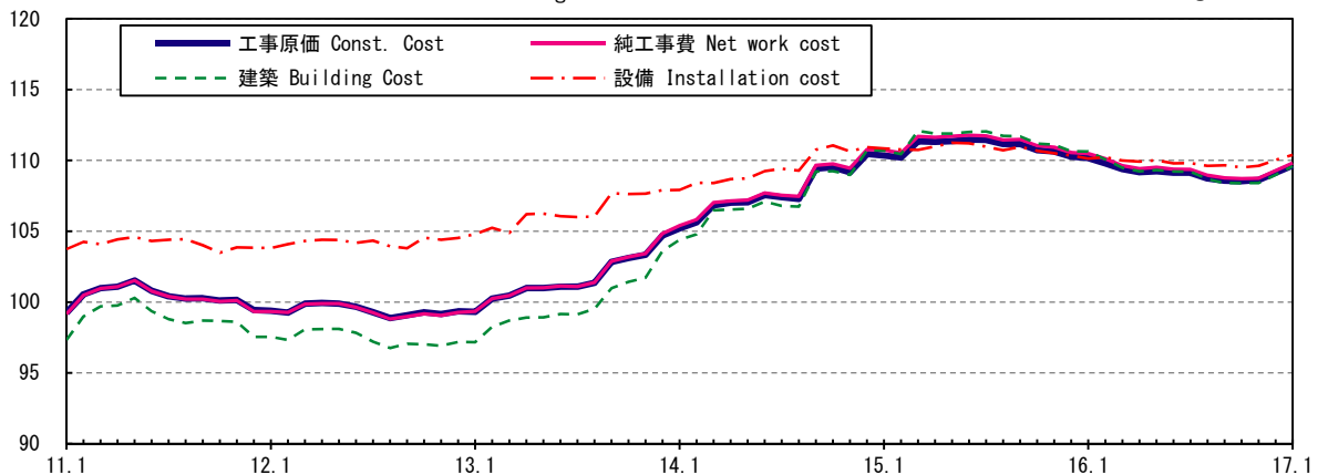
図-2 No. 6 事務所 S 平成17年平均=100 fig. 2 Office 2005 average=100
