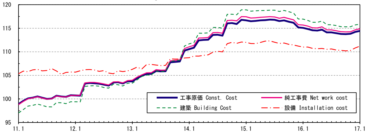
図-1 No. 2 集合住宅 RC 平成17年平均=100 fig. 1 Condominium 2005 average=100
