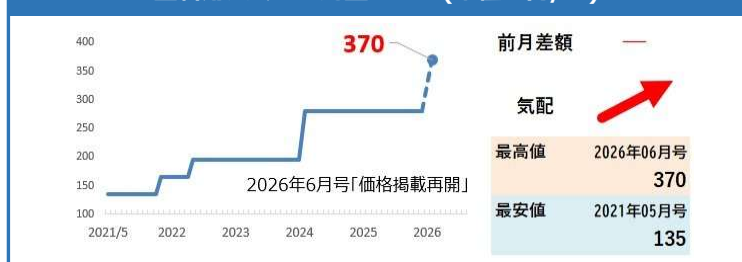
塗料用シンナー 比重0.79 (単位：円/ℓ)
